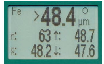
Statistik-Funktionen
