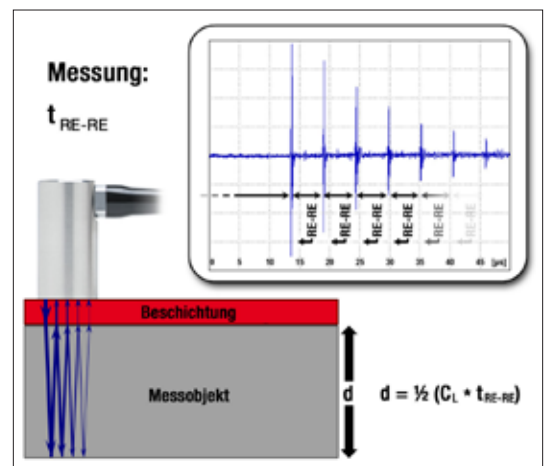
Das Messprinzip bei beschichtetem Material: Bestimmung der Laufzeit aufeinanderfolgender Rückwändechos (RE-RE-Modus)
