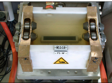
Prüfkammer für Wanddickenmessung und Dopplungsprüfung
