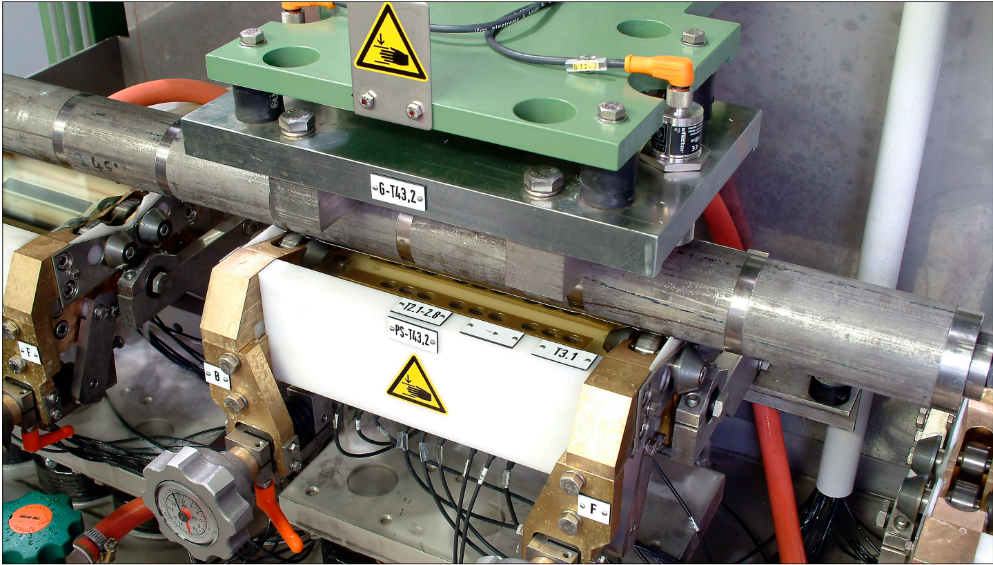
Die Kalibrierung des Prüfsystems wird mit Rohren durchgeführt, die künstliche Fehler aufweisen. Längs- und Quernuten auf der inneren und äußeren Rohroberfläche werden zur Kalibrierung der Winkelfunktionen verwendet. Kreisscheibenreflektoren oder Nuten können zur Kalibrierung der Senkrechtprüfköpfe verwendet werden.
