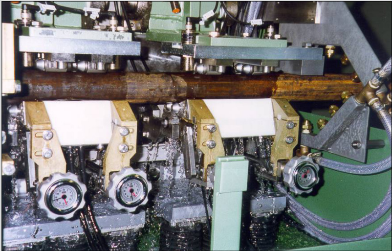
Ansicht von zwei Prüfkammern für die Ultraschallprüfung mit Pfützentechnik (Prüfköpfe unter dem Rohr in der wassergefüllten Kammer). Das gezeigte Prüfsystem verwendet eine Kammer für die Erkennung von Längsfehlern. Die zweite Kammer wird für Quer- oder Schrägfehler verwendet. Die Handräder dienen zur Einstellung der Prüfkopf-Einschallwinkel.
