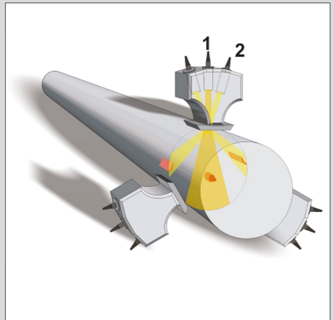
Prüfkopfhalter für runde Knüppel mit einem Senkrechtprüfkopf. Zwei optionale Prüfköpfe werden für die Winkleinschallung verwendet.
