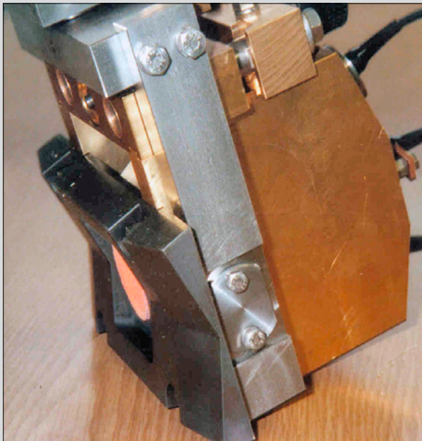
Prüfkopfhalter für runde Knüppel mit einem Senkrechtprüfkopf. Zwei optionale Prüfköpfe werden für die Winkleinschallung verwendet.
