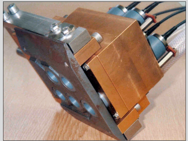
Prüfkopfhalter für quadratische Knüppel. Die Ultraschallkopplung wird durch geführte Wasserstrahlen (Squirtertechnik) erreicht.
