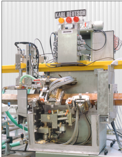
ECHOGRAPH-KNPS-Prüfsystem
