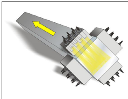
Prüfprinzip für quadratische Knüppel (28 Prüfköpfe)
