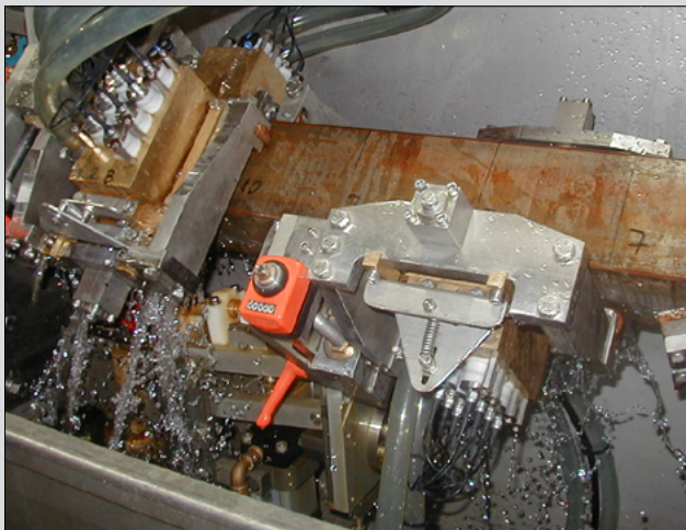
Vier Prüfkopfhalter für quadratische Knüppel, jeder Träger mit sieben Prüfköpfen und Positionierung von allen vier Seiten. Die Führung wird durch Führungsrollen und Hartmetallkufen erreicht.
