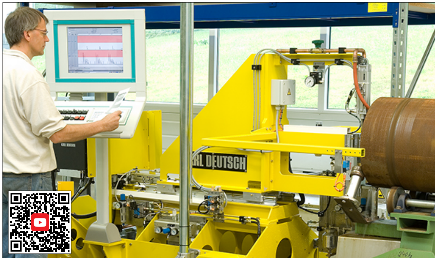
Eingabe der Prüfparameter und Überprüfung der Kalibrierung des Prüfsystems
